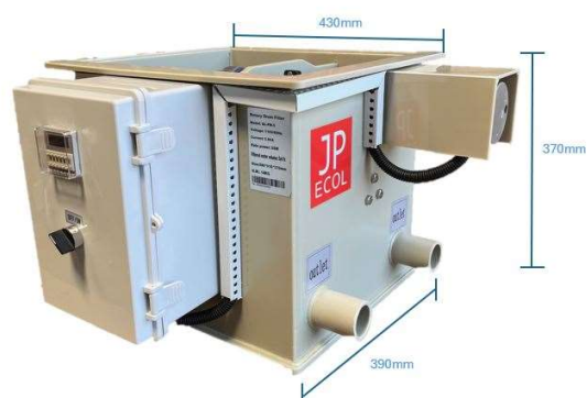
強制濾過機本体(PM05)
